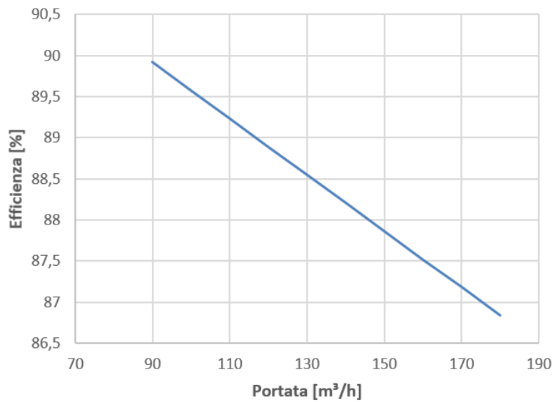
Curva di efficienza RDE 018
