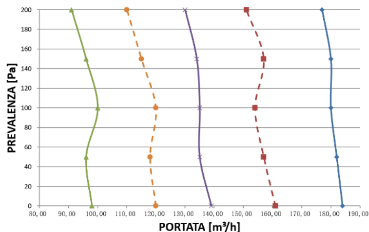
Curva portata – prevalenza RDE 018
