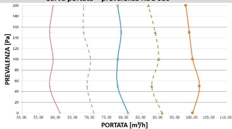
Curva portata – prevalenza RDE 010
