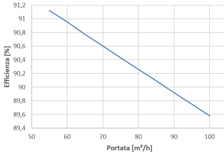
Curva di efficienza RDE 018
