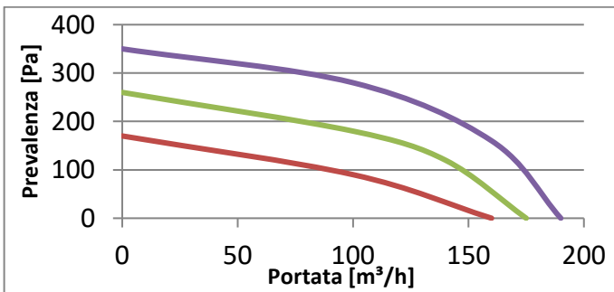
Curva portata – prevalenza RCE 016
