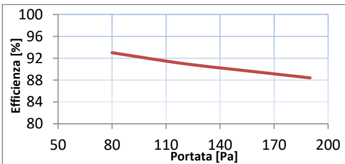
Curva di prestazione RCE 016
